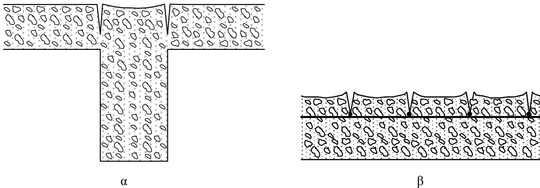
Σχήμα 2: Ρηγμάτωση από καθίζηση σκυροδέματος σε πλαστική κατάσταση
