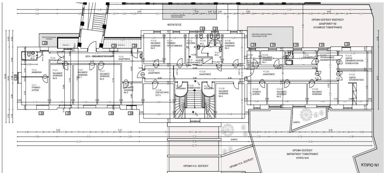
Σχεδίο 1. Κάτοψη Ορόφου Υ1 Κτιρίου της ΩΡΛ-ΟΦΘ/ΚΗΣ-Οδοντιατρικής Κλινικής
