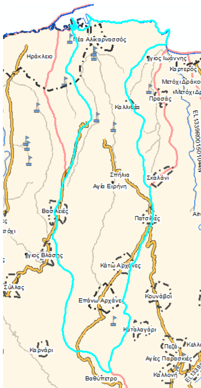
Εικόνα 1: Η Περιοχή Υδραυλικής μελέτης του Σιλαμιανού ρέματος
