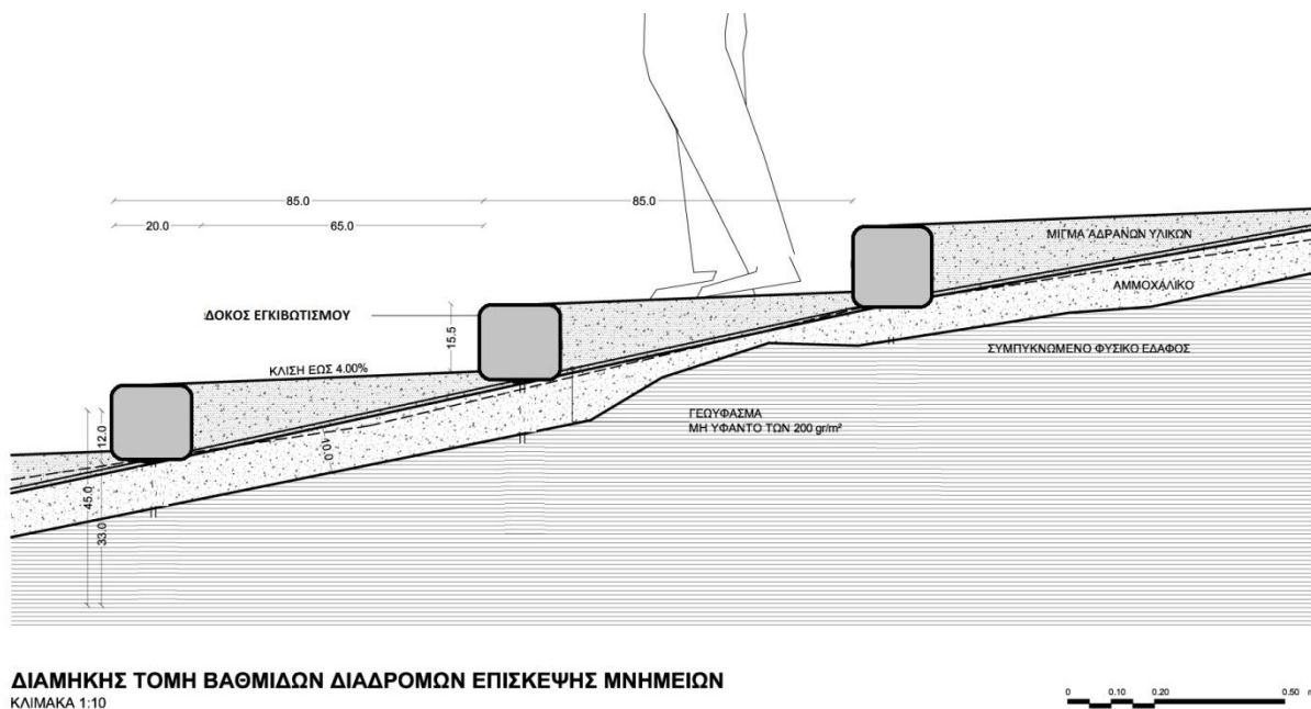
Εικ. 6: Αποκατάσταση Βαθμίδων: ενδεικτική τομή βαθμιδωτής διαμόρφωσης - εγκιβωτισμός παλιού κονιάματος
