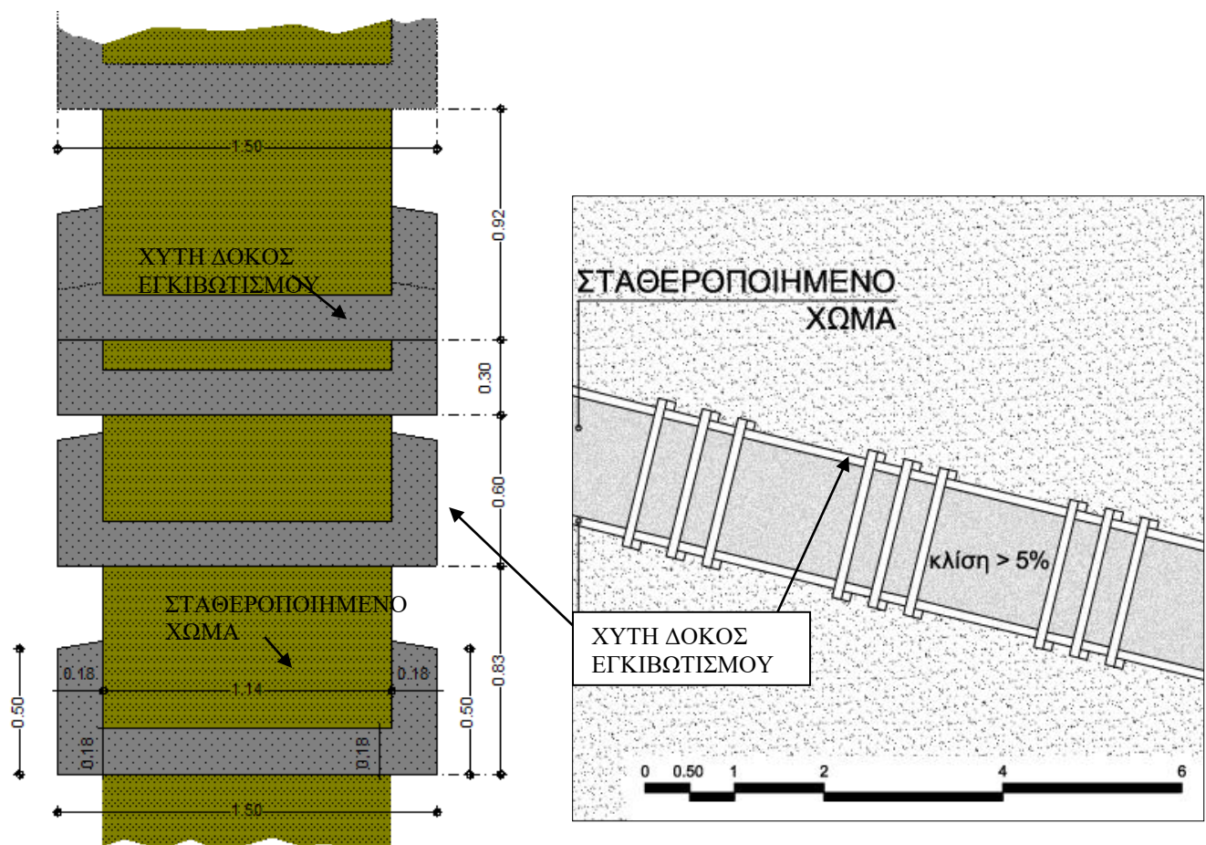
Εικ. 5: Αποκατάσταση Βαθμίδων: ενδεικτική κάτοψη βαθμιδωτής διαμόρφωσης - εγκιβωτισμός παλιού κονιάματος
