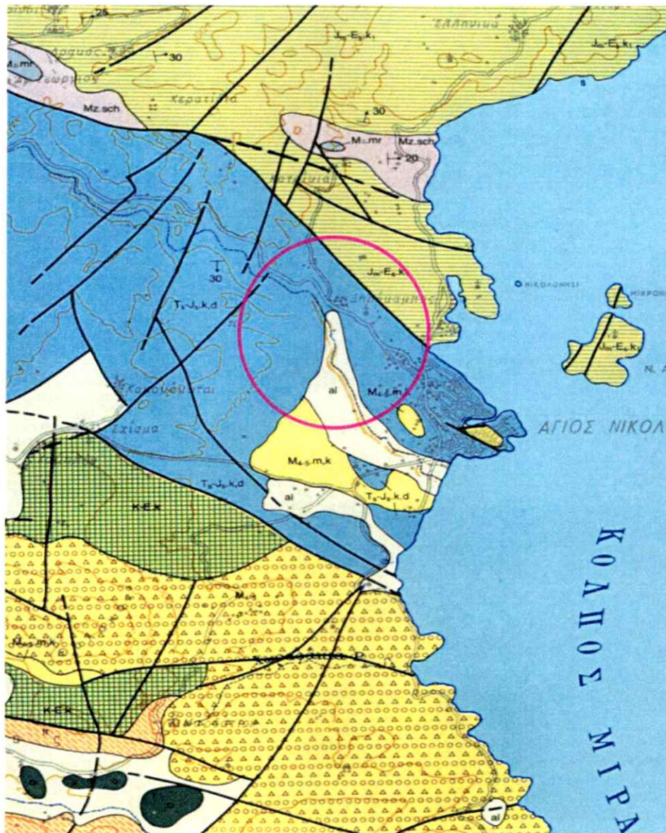
Γεωλογικός χάρτης περιοχής της μελέτης (από ΙΓΜΕ, Φύλλο ΑΓ. ΝΙΚΟΛΑΟΣ, κλίμακα 1:50.000)
