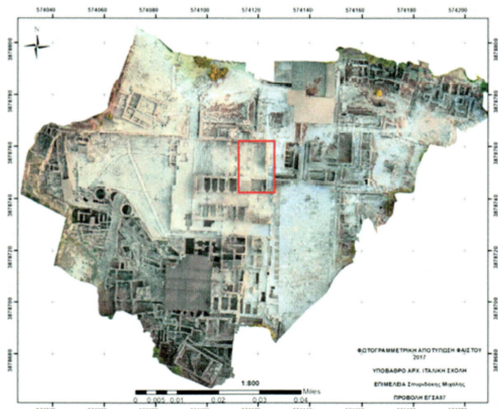
Κάτοψη μινωικού ανακτόρου της Φαιστού. Με κόκκινη σήμανση η περιοχή επέμβασης (φωτογραμμετρία, Μιχάλης Σπυριδάκης).
