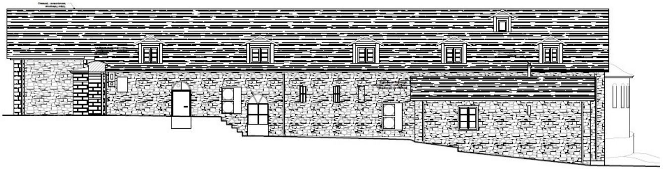
ΝΟΤΙΑ ΟΨΗ ΚΑΙΜΑΚΑ 1:75
