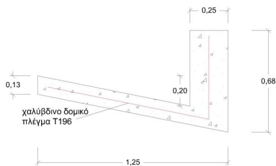
Τυπική διατομή τάφρου
