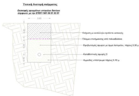
Τυπική διατομή σκάμματος
