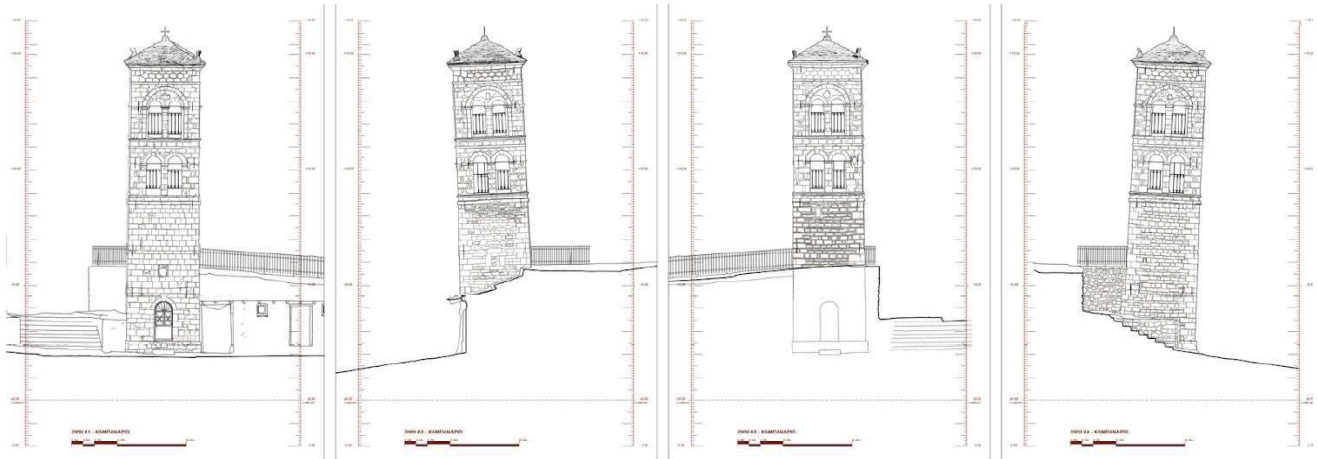
Αποτύπωση υπάρχουσας κατάστασης: Ανατολική, Βόρεια, Δυτική και Νότια Όψη (Τ. Κουιμπζόγλου, 2022)
