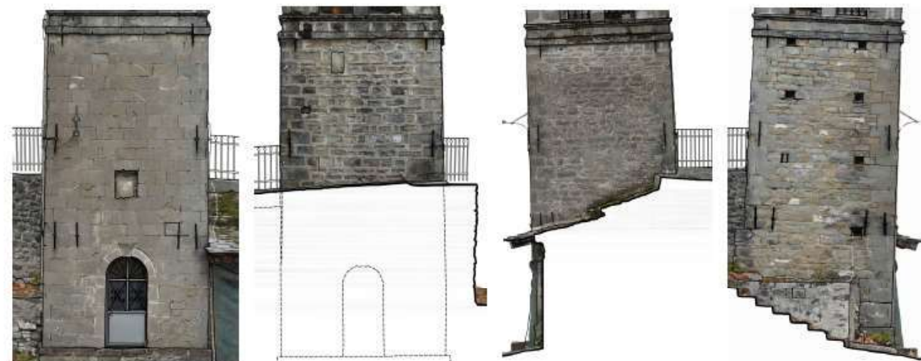
Κάτω τμήμα κωδωνοστασίου, όψεις διαδοχικά: Ανατολική, Δυτική, Βόρεια και Νότια (Τ. Κουιμπζόγλου, 2022)
