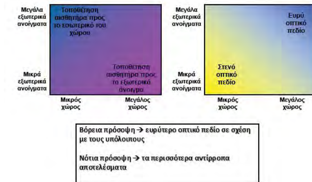
Σχήμα 5.3. Τοποθέτηση και πεδίο όρασης αισθητήρων φωτισμού σε συνάρτηση με το μέγεθος του χώρου και των εξωτερικών ανοιγμάτων
