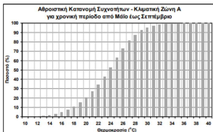
Διάγραμμα 6.1 Αθροιστική κατανομή συχνοτήτων θερμοκρασίας εξωτερικού αέρα για χρονική περίοδο από Μάιο έως Σεπτέμβριο για την Κλιματική Ζώνη Α.
